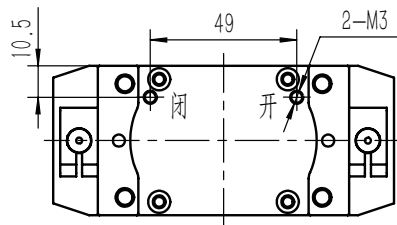
B底部通气款底部气孔尺寸示意
